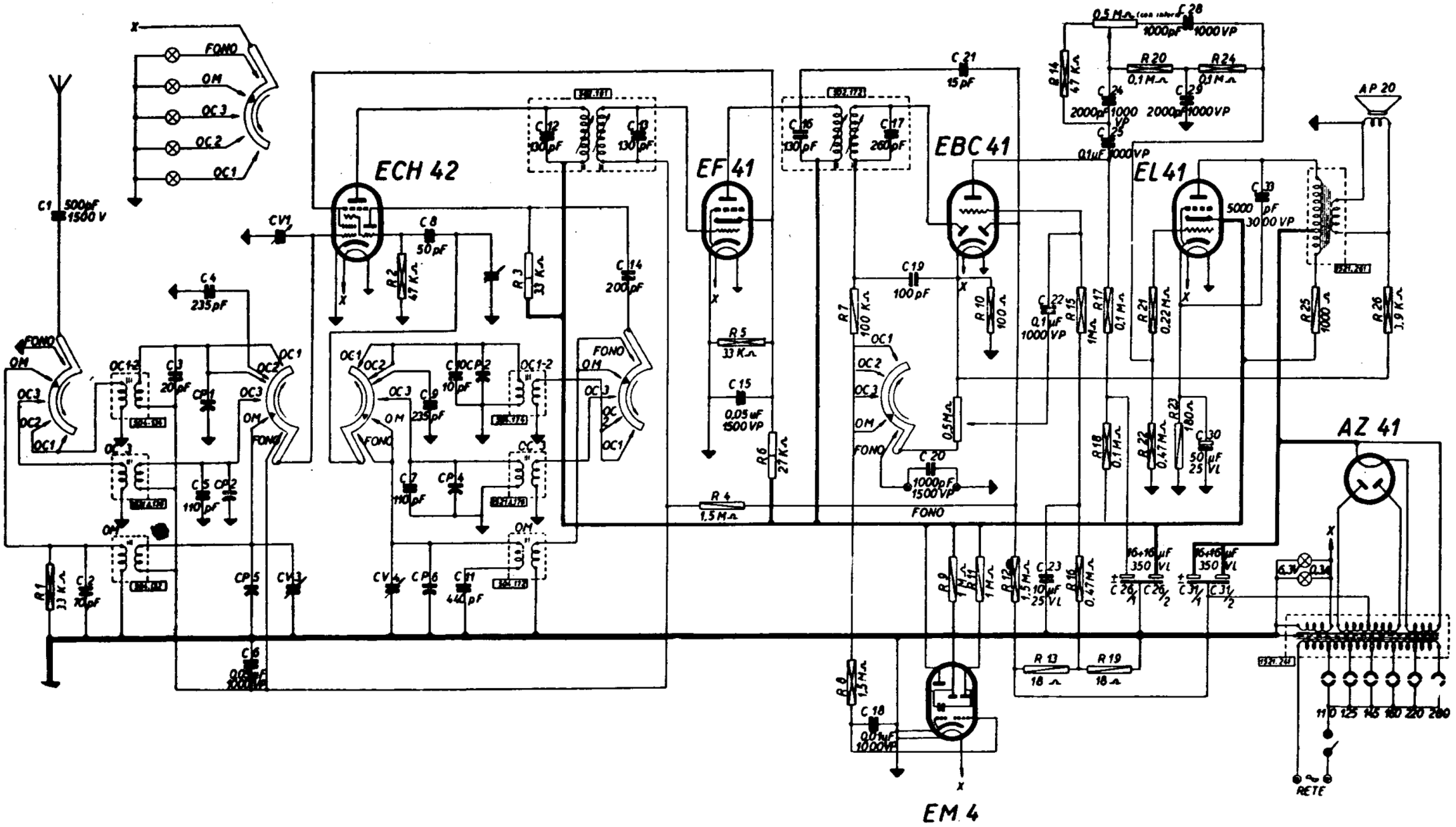
VOCE DEL PADRONE - Mod. 1525. Onde medie e tre gamme espanse onde corte. Media frequenza 465 kc/s. Potenza indistorta di uscita 3 watt. Consumo 45 watt.
